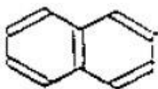
Naftalin
